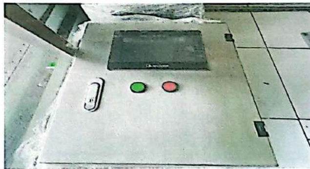
Gambar 1. 4 Panel PLC dengan HMI application
