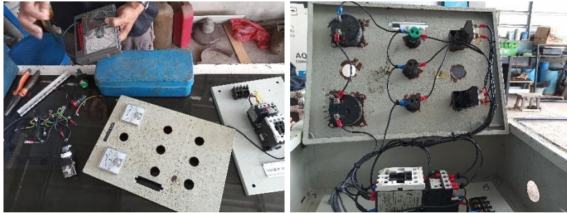
Gambar 2. 6 Perbaikan Panel Pompa 3 Phase
