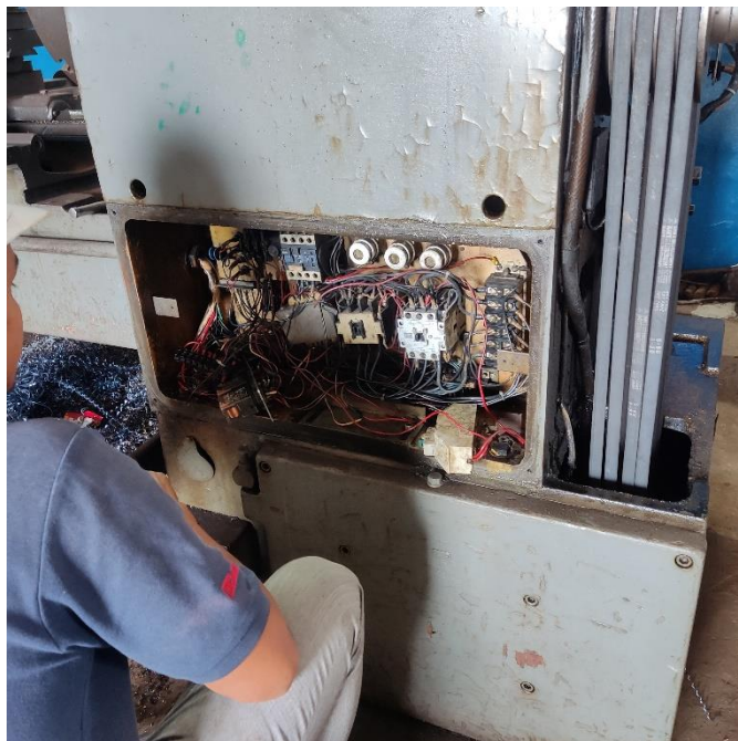
Gambar 2.4 Proses pemeriksaan dan perbaikan kerusakan pada mesin bubut.
