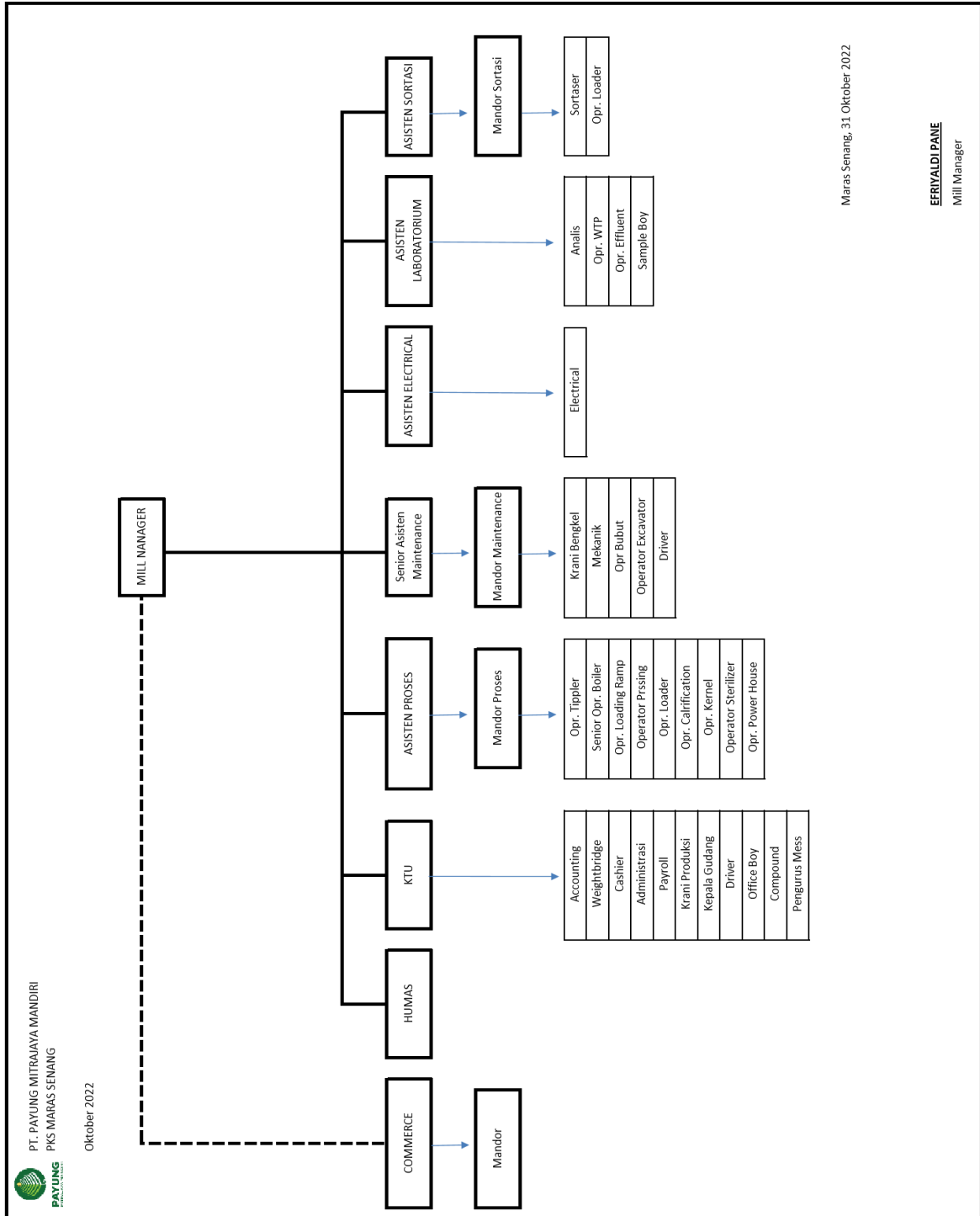
Gambar 1.3 Struktur organisasi
