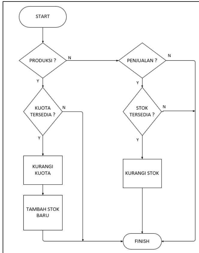
Gambar 2.3 Flowchart Produksi dan Penjualan
