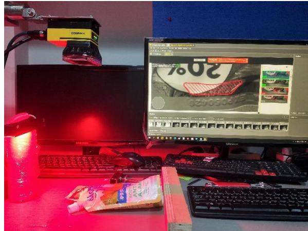
Gambar 2.2 Inspection Gelembung pada produk BioDef menggunakan kamera ISD 905M (Deep Learning)
