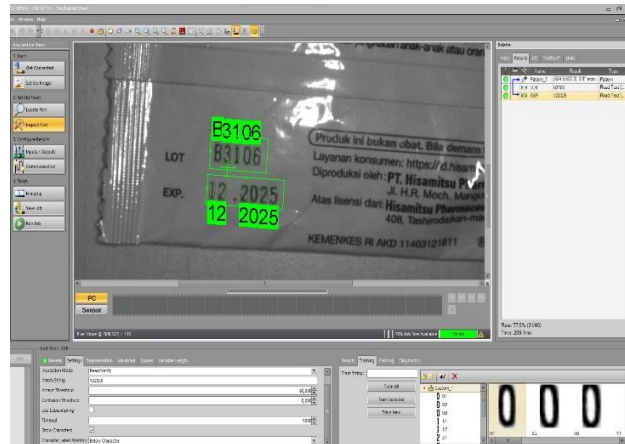
Gambar 2.3 Inspection posisi label dan expired date pada produk ByeBye-FEVER
