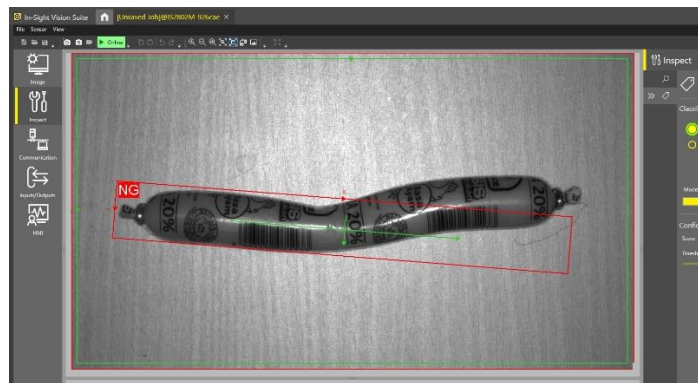
Gambar 2.1 Inspection bentuk sosis menggunakan software In Sight Vision Suite, Camera In Sight 2802M
