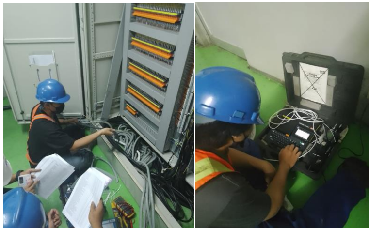
Gambar 2.9 Pengerjaan Terminasi Panel MCC
